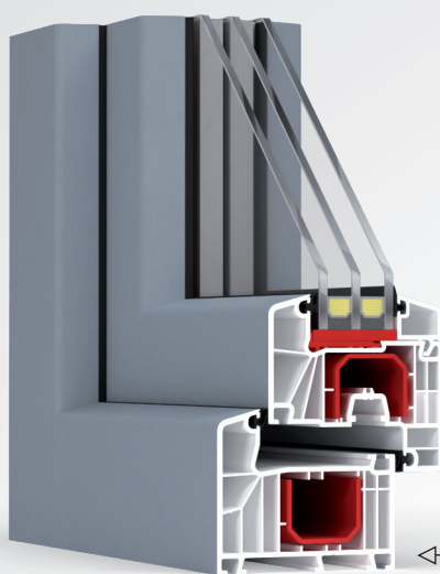
Skrzydło i rama ideal 7000 AP 34
